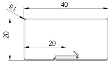
Tube 20x40
