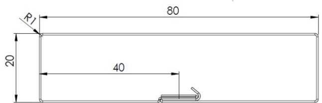
Tube 20x80
